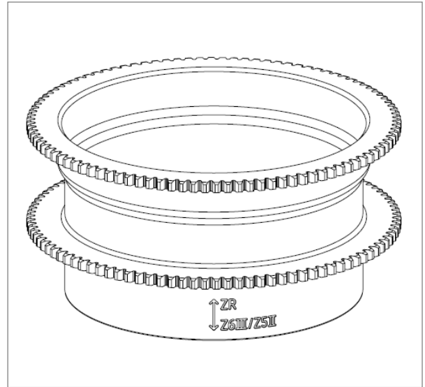
Z1430-ZII Zoom Gear
